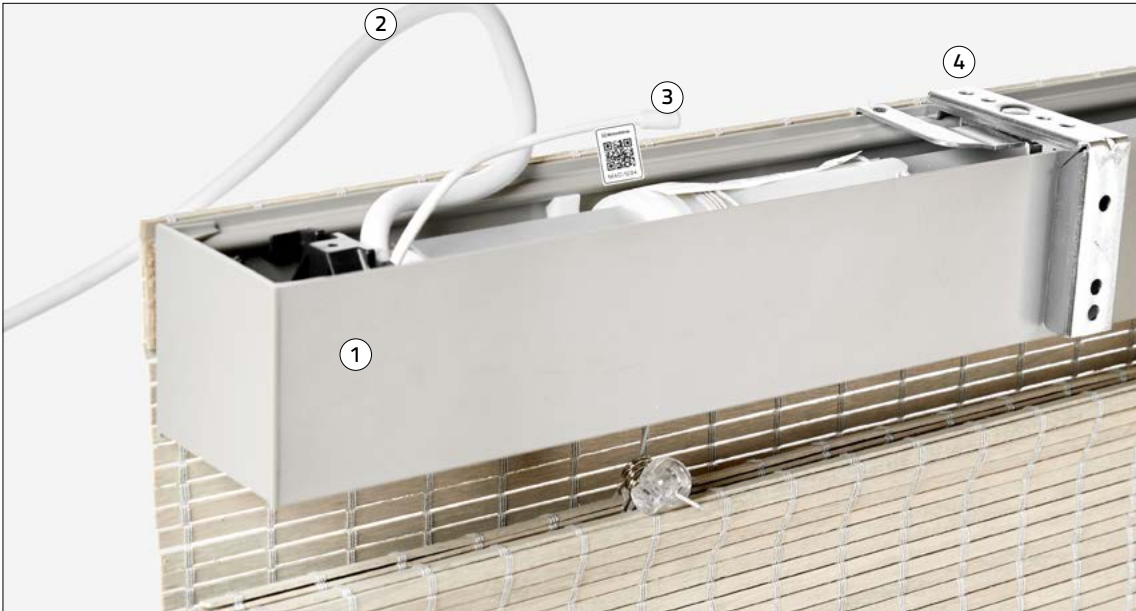
Roman blind: CM-09-QC radio motor
